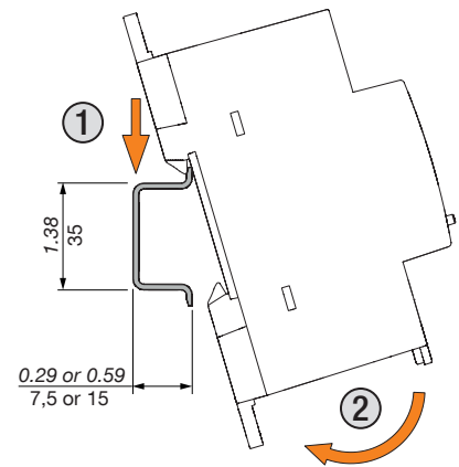
DIN rail
