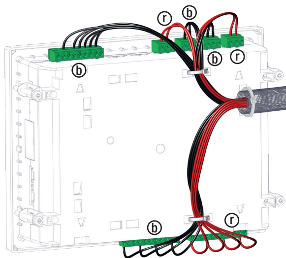
Right side hinge door
